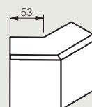
CL outside lid 45° bend
