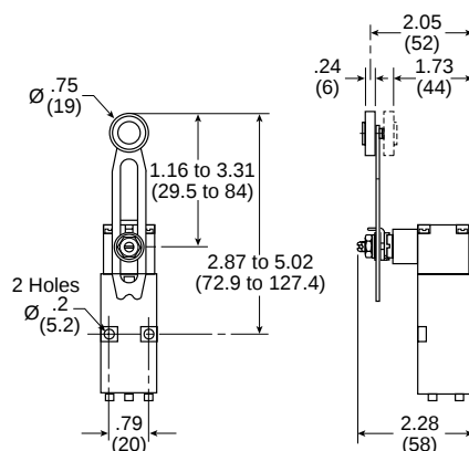
PXCK2110541, PXCK2210541
