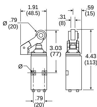
PXCK21121, PXCK22121
