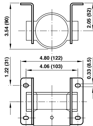
F22 Bracket (18-001-962)
