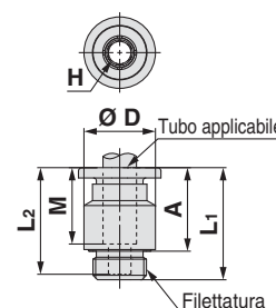
Dimensioni anello di rilascio
