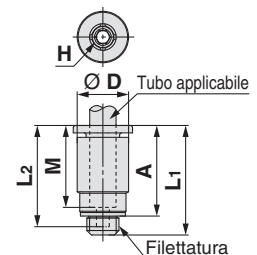
Dimensioni anello di rilascio
