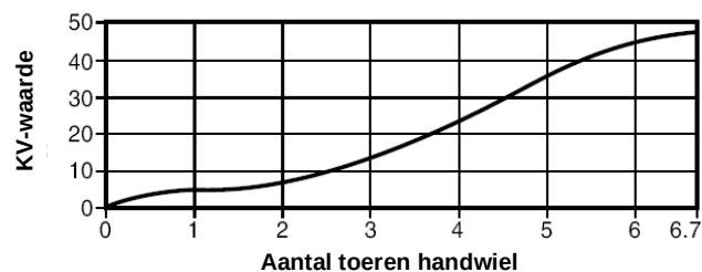
BSAT - DN80
