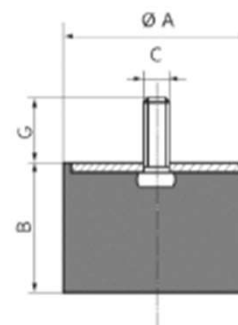
Type D Block 1 Stud
