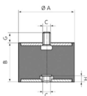
Type B 1 Stud
