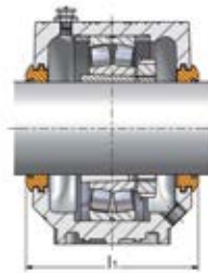
Labyrinthdichtung SC..LA
