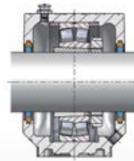
Filzstreifendichtung SC..FS
