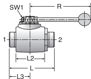
DN32 - DN40
